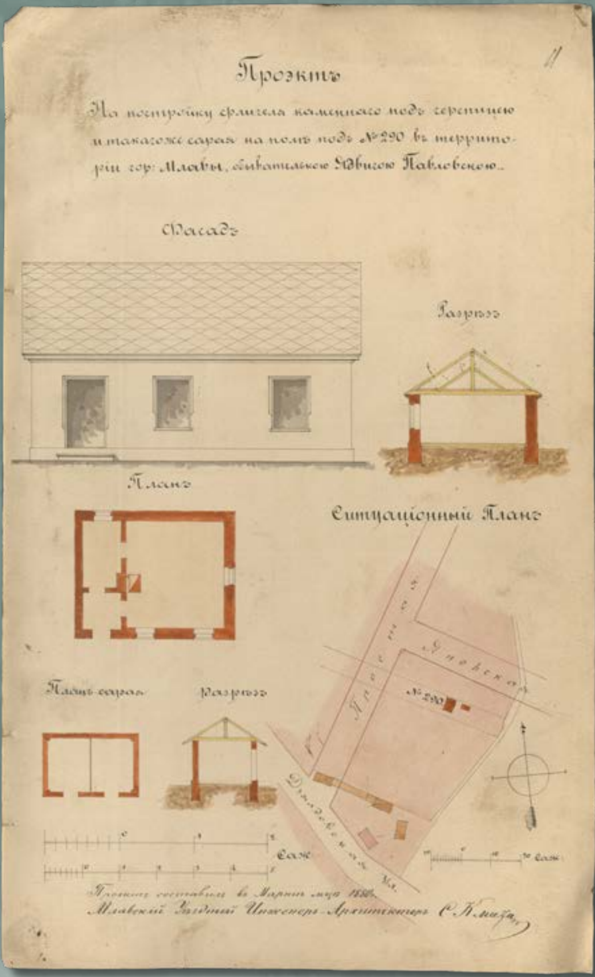
Projekt murowanej oficyny krytej dachówką oraz składu na drewno w nieruchomości pod numerem 290 w Mławie, wł. Jadwiga Pawłowska, 1880 rok (źródło: Archiwum Państwowe w Płocku, Płocki Rząd Gubernialny, sygn. 3160, k. 11)
