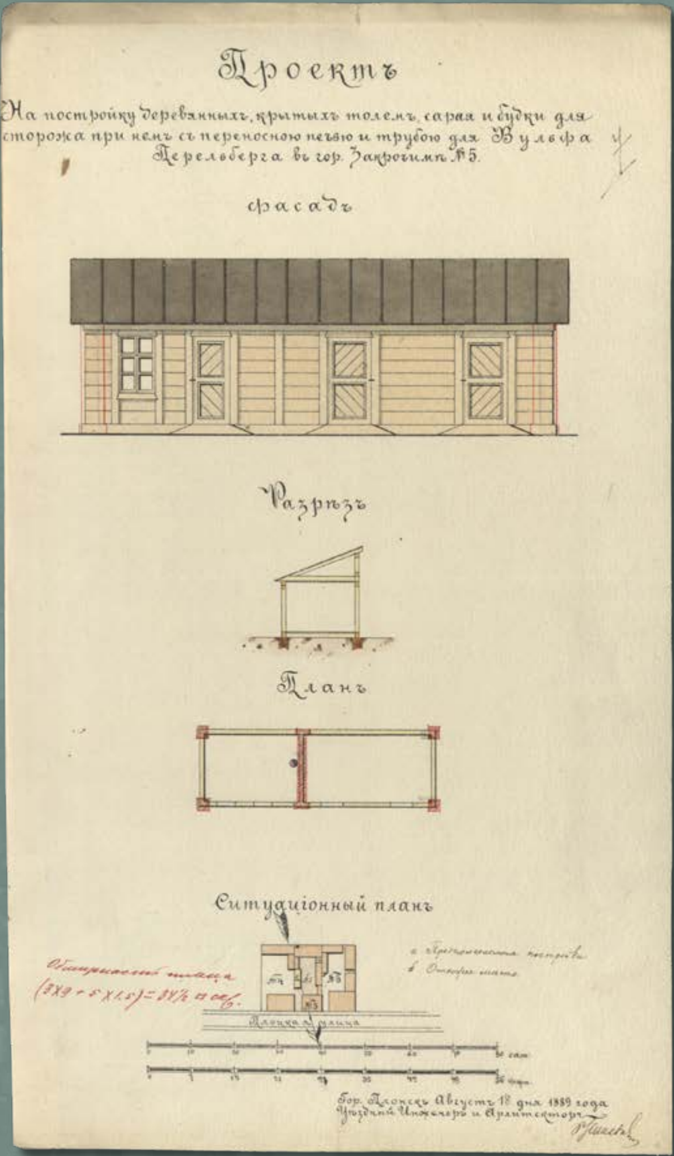
Projekt drewnianych krytych papą szopy i budki dla stróża w nieruchomości numer 5 przy ulicy Płockiej w Zakroczymiu, wł. Wulf Perelberg, 1889 rok (źródło: Archiwum Państwowe w Płocku, Płocki Rząd Gubernialny, sygn. 3210, k. 7)
