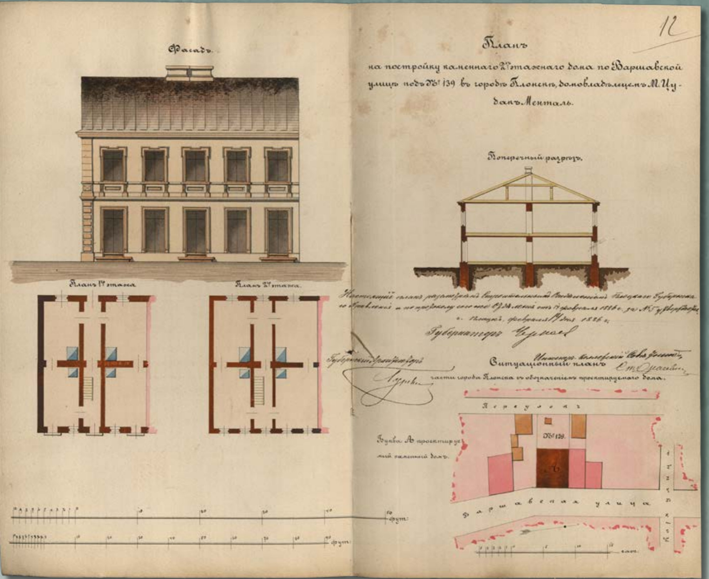
Projekt murowanego dwupiętrowego domu w nieruchomości numer 139 przy ulicy Warszawskiej, wł. Cudek Mental, 1886 rok (źródło: Archiwum Państwowe w Płocku, Płocki Rząd Gubernialny, sygn. 3197, k. 11-12)
