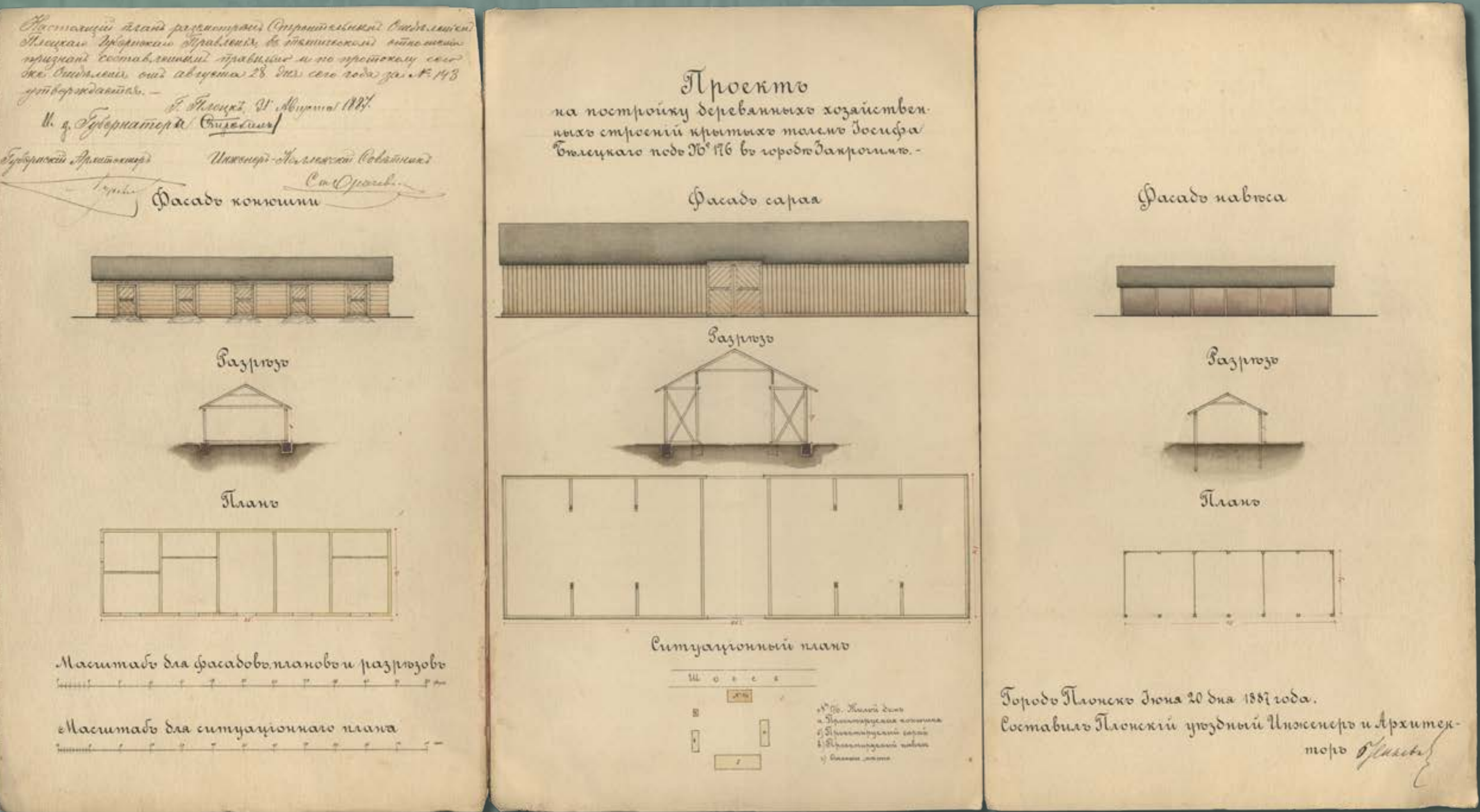
Projekt drewnianych gospodarczych budynków krytych papą w nieruchomości numer 176 w Zakroczymiu, wł. Józef Bielecki, 1887 rok (źródło: Archiwum Państwowe w Płocku, Płocki Rząd Gubernialny, sygn. 3200)
