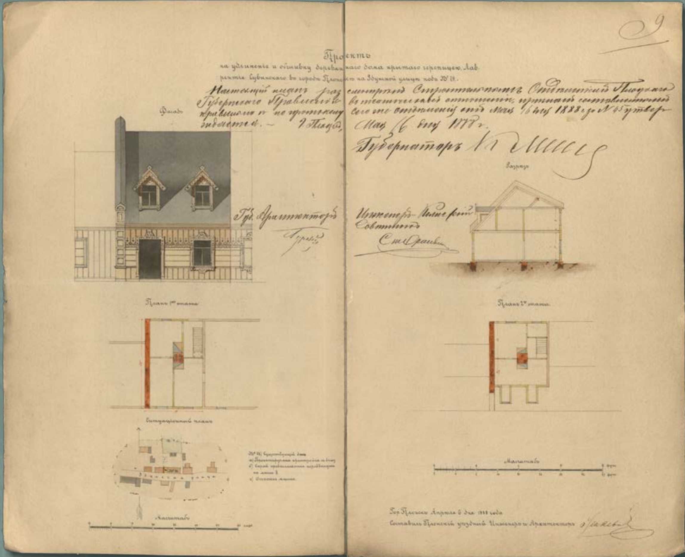
Projekt przebudowy drewnianego domu krytego dachówką w nieruchomości numer 79 przy ulicy Zduńskiej, wł. Wawrzyniec Suwiński, 1888 rok (źródło: Archiwum Państwowe w Płocku, Płocki Rząd Gubernialny, sygn. 3204, k. 9)
