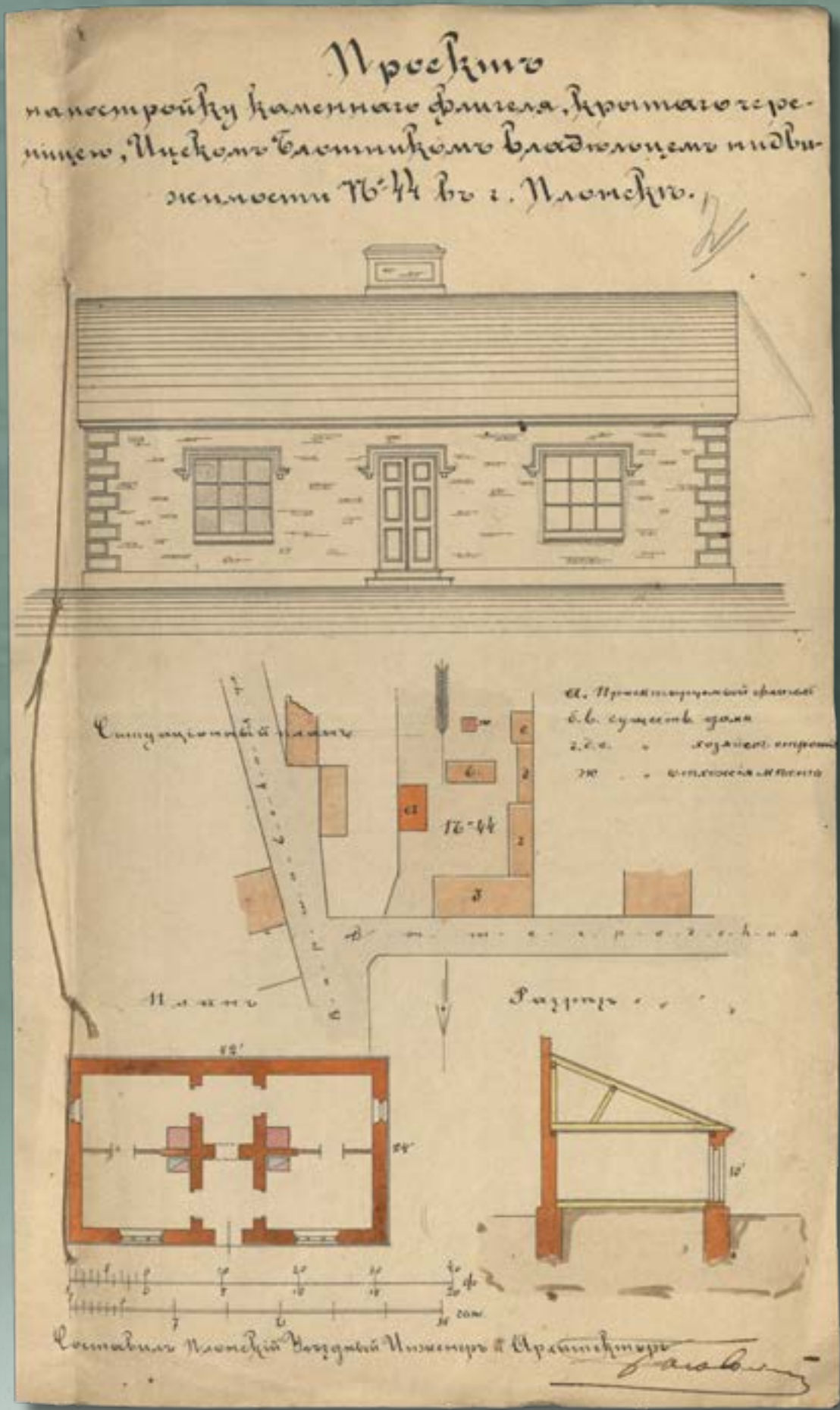
Projekt murowanej oficyny krytej dachówką w nieruchomości numer 44 przy ulicy Wyszogrodzkiej w Płońsku, wł. Icek Błotnik, 1894 rok (źródło: Archiwum Państwowe w Płocku, Płocki Rząd Gubernialny, sygn. 3231, k. 2)
