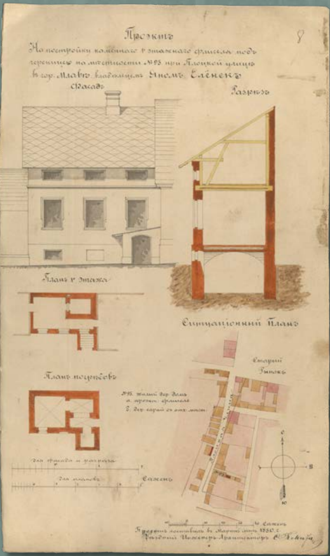
Projekt murowanej jednopiętrowej oficyny krytej dachówką w nieruchomości numer 95 przy ulicy Płockiej w Mławie, wł. Jan Jelonek, 1880 rok (źródło: Archiwum Państwowe w Płocku, Płocki Rząd Gubernialny, sygn. 3160, k. 8)
