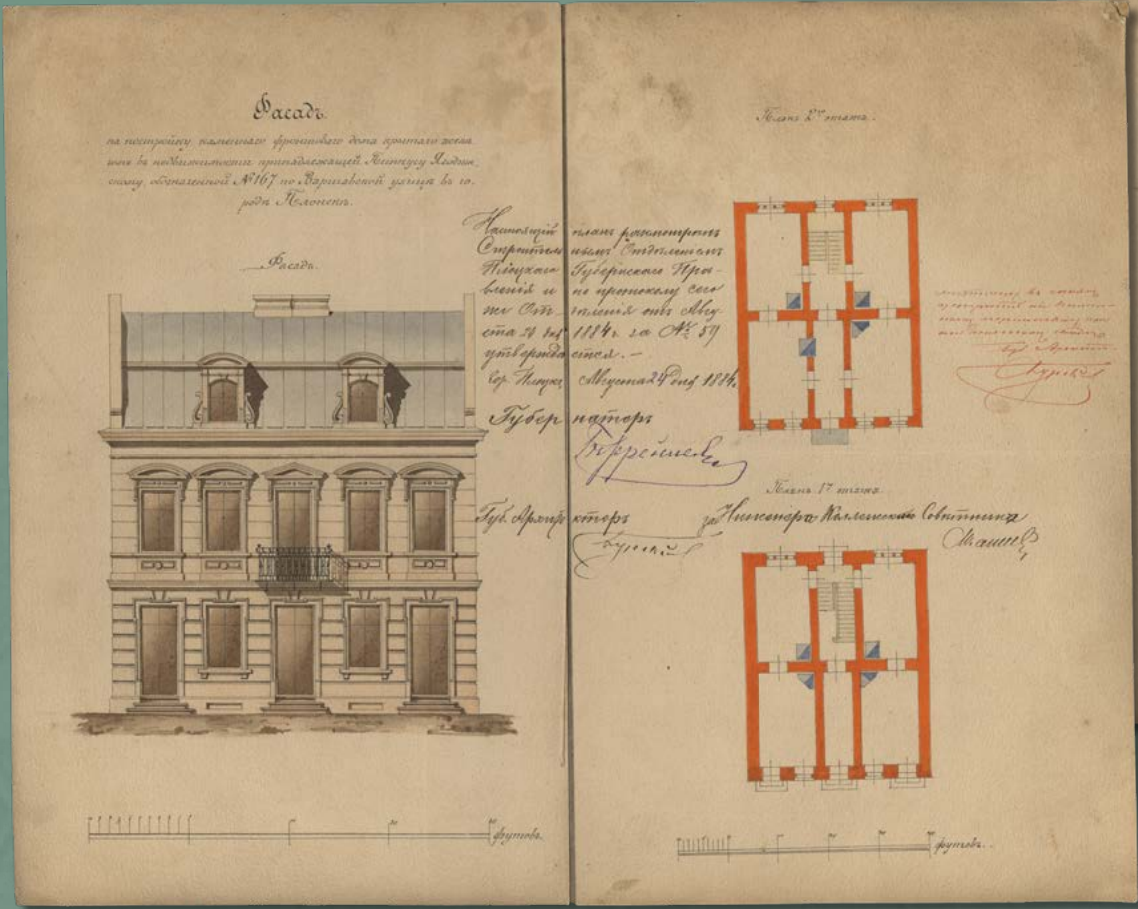
Projekt murowanego frontowego domu krytego blachą żelazną w nieruchomości numer 167 przy ulicy Warszawskiej w Płońsku, wł. Pinkus Jagodziński, 1884 rok (źródło: Archiwum Państwowe w Płocku, Płocki Rząd Gubernialny, sygn. 3190, k. 30)
