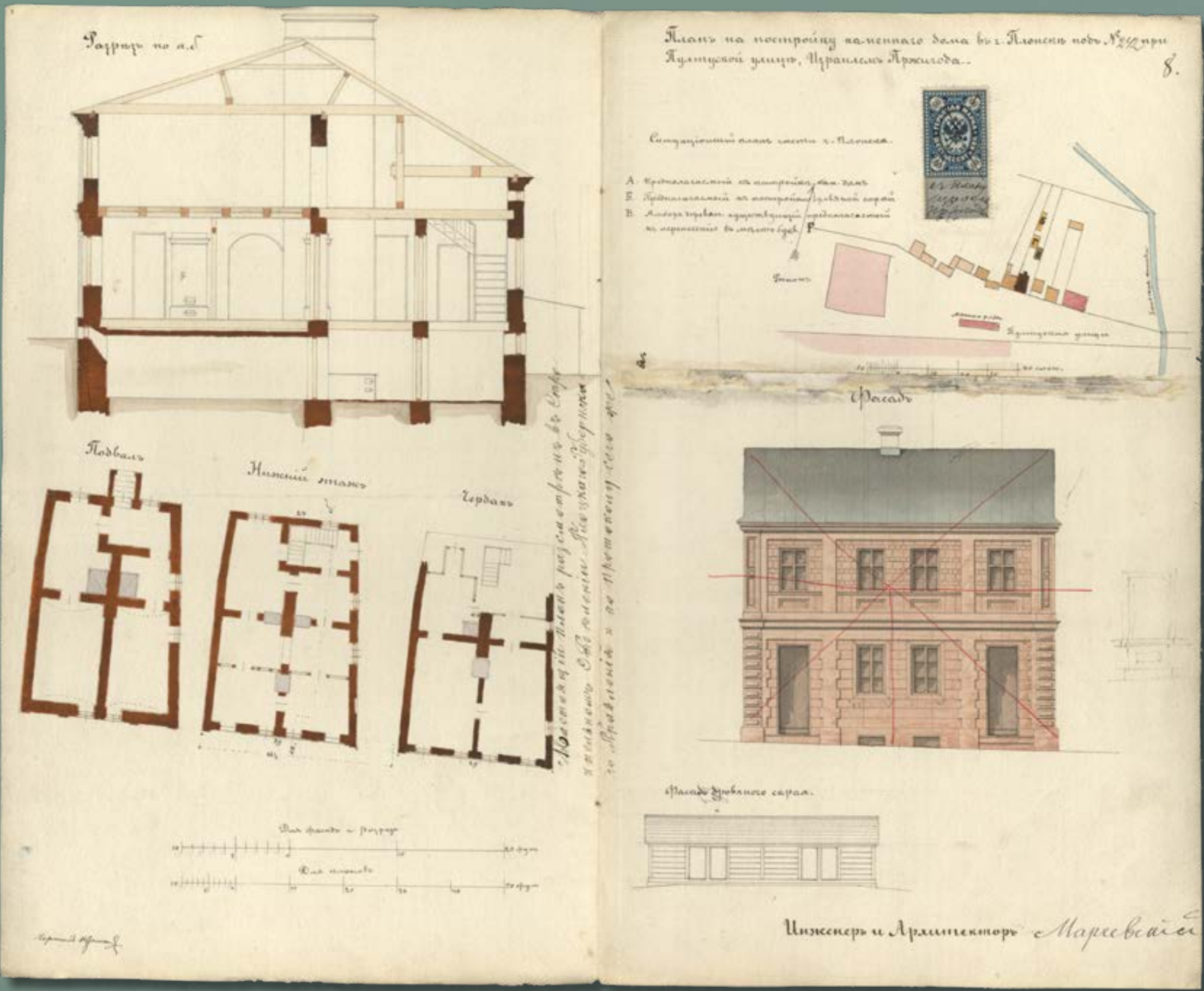
Projekt murowanego domu w nieruchomości numer 242 przy ulicy Pułtuskiej w Płońsku, wł. Izrael Przygoda, 1882 rok (źródło: Archiwum Państwowe w Płocku, Płocki Rząd Gubernialny, sygn. 3175, k. 7–8)
