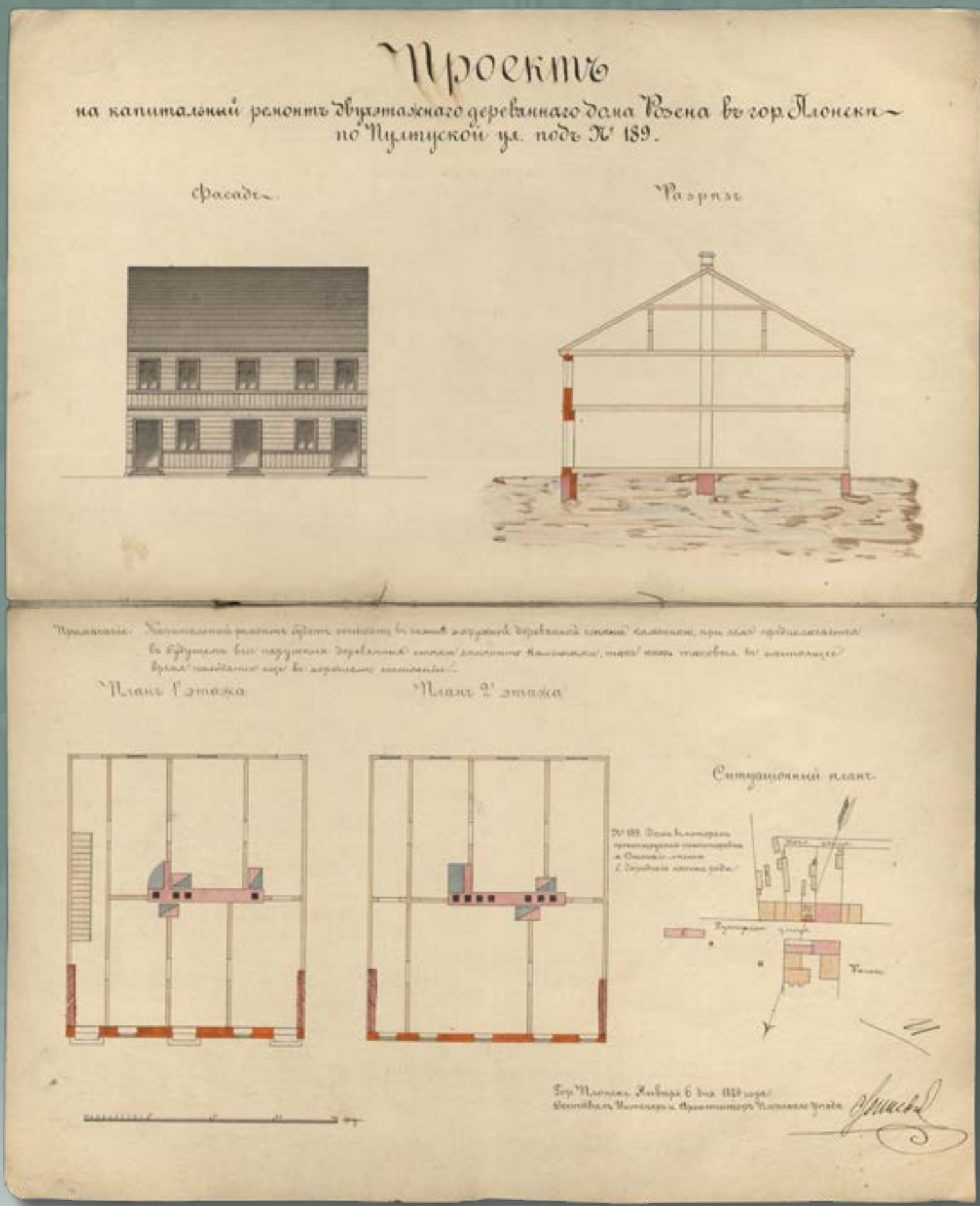
Projekt kapitalnego remontu drewnianego domu przy ulicy Pułtuskiej numer 189 w Płońsku, wł. Lejb Rozen, 1889 rok (źródło: Archiwum Państwowe w Płocku Płocki Rząd Gubernialny, sygn. 3206, k. 10-11)
