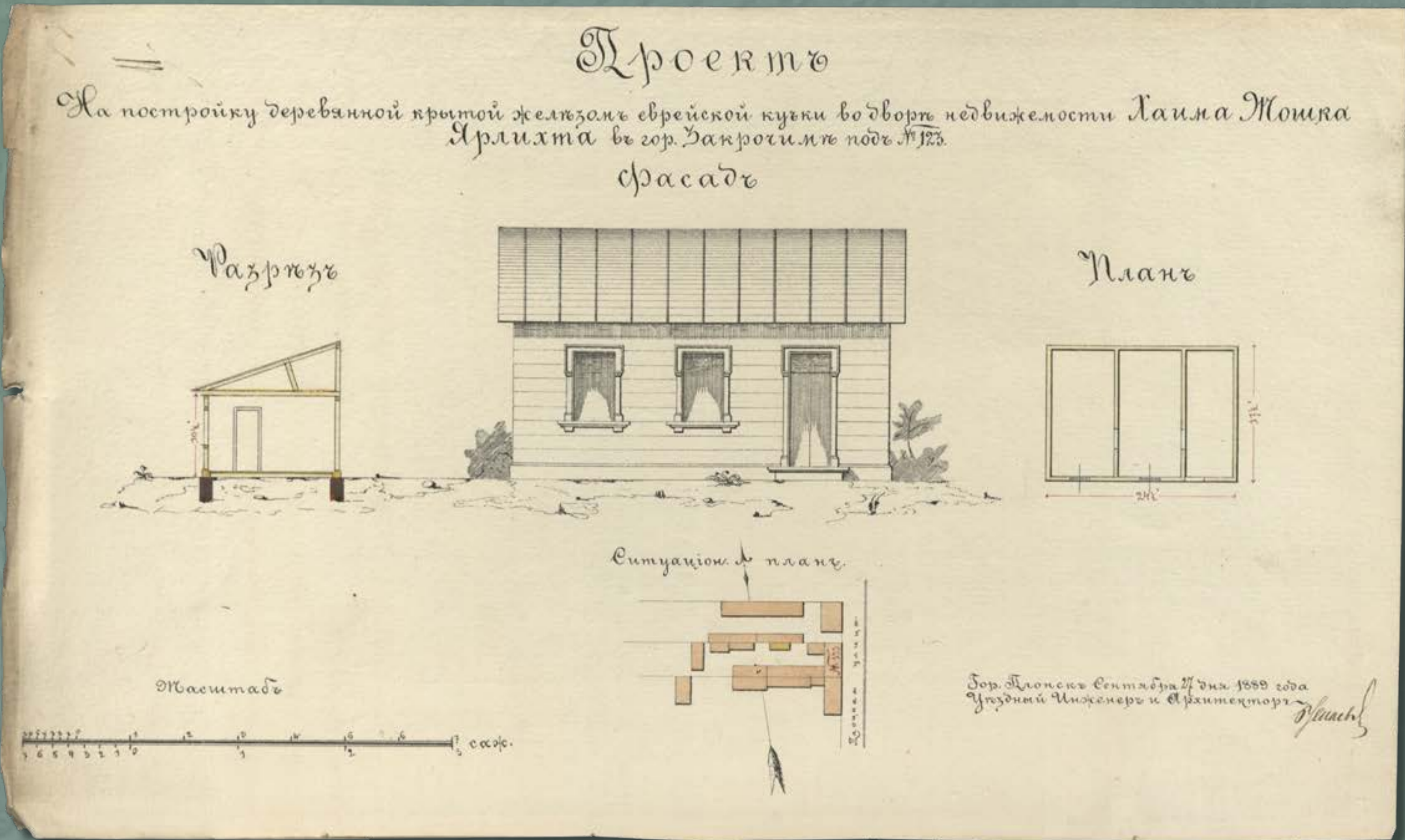
Projekt drewnianej krytej blachą żelazną kuczki w podwórzu nieruchomości numer 123 przy ulicy Płockiej w Zakroczymiu, wł. Chaim Moszek Jarlicht, 1889 rok (źródło: Archiwum Państwowe w Płocku, Płocki Rząd Gubernialny, sygn. 3210)
