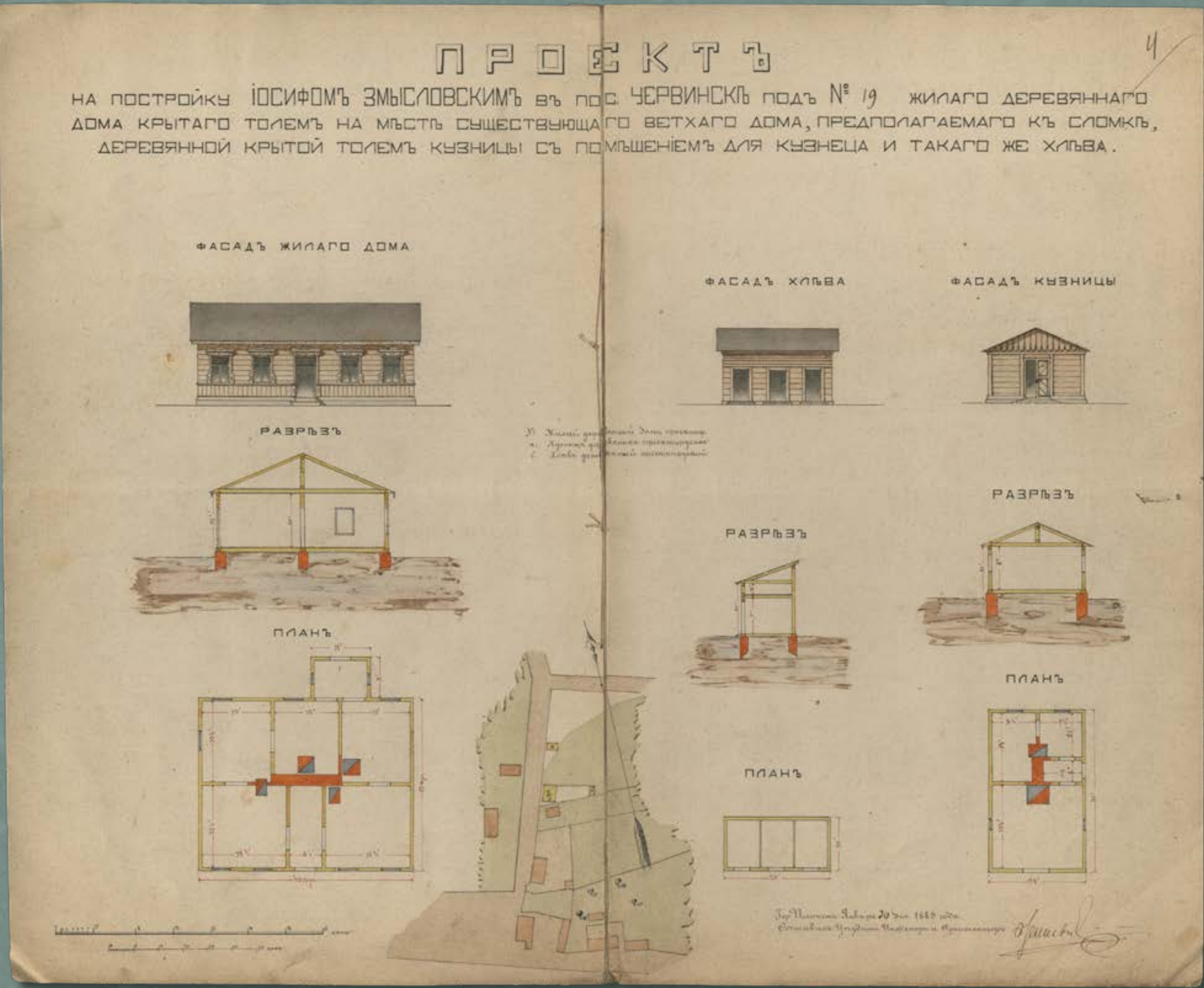
Projekt drewnianego domu mieszkalnego krytego papą, drewnianej kuźni krytej papą z pomieszczeniem dla kowala i chlewu w nieruchomości pod numerem 19 w Czerwińsku, wł. Józef Zmysłowski, 1889 rok (źródło: Archiwum Państwowe w Płocku, Płocki Rząd Gubernialny, sygn. 3208, k. 4)
