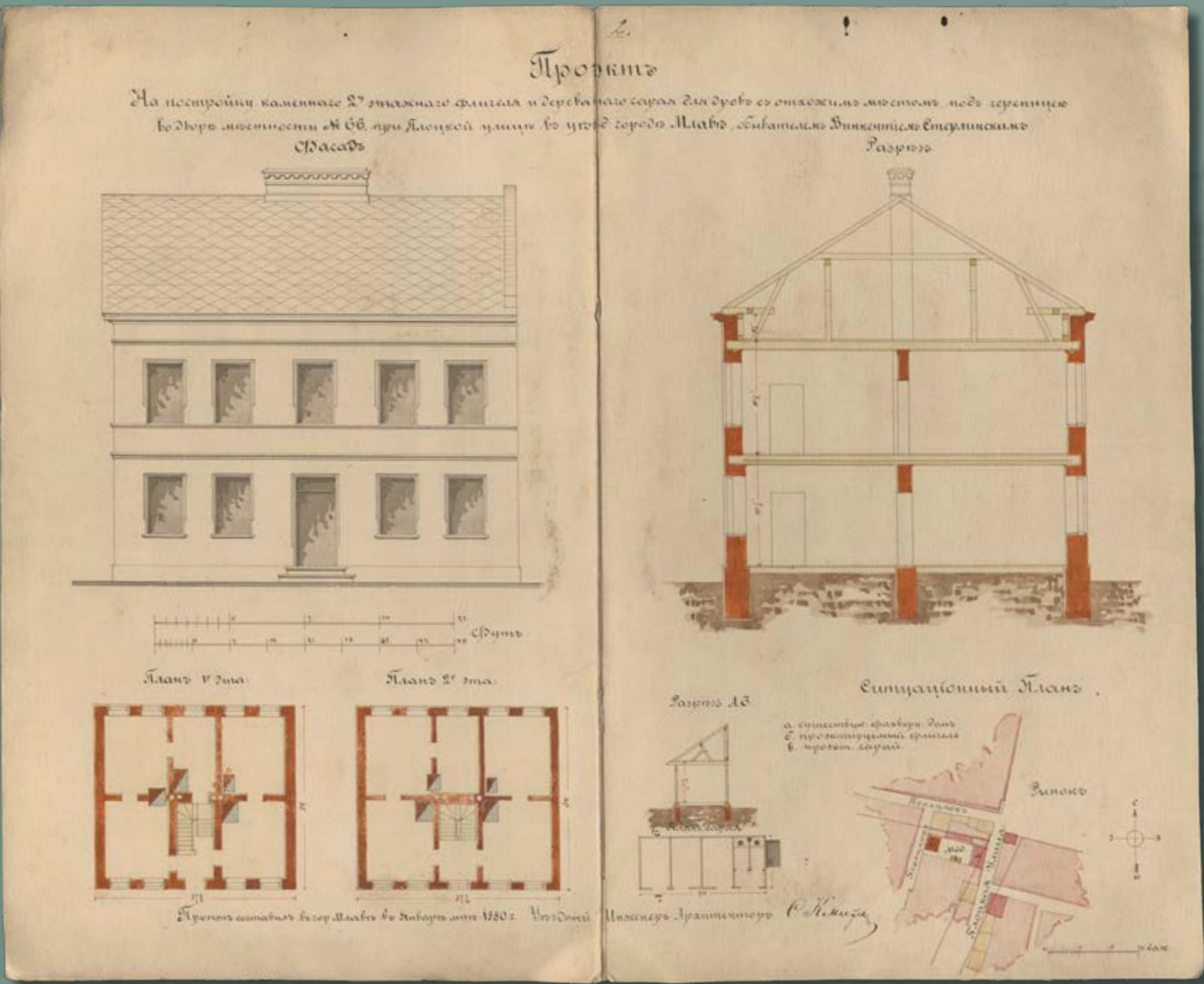
Projekt murowanej dwupiętrowej oficyny i drewnianego składu na drewno z ustępami krytych dachówką w podwórzu nieruchomości pod numerem 66 przy ulicy Płockiej w Mławie, wł. Wincenty Sterliński, 1880 rok (źródło: Archiwum Państwowe w Płocku, Płocki Rząd Gubernialny, sygn. 3160, k. 2)
