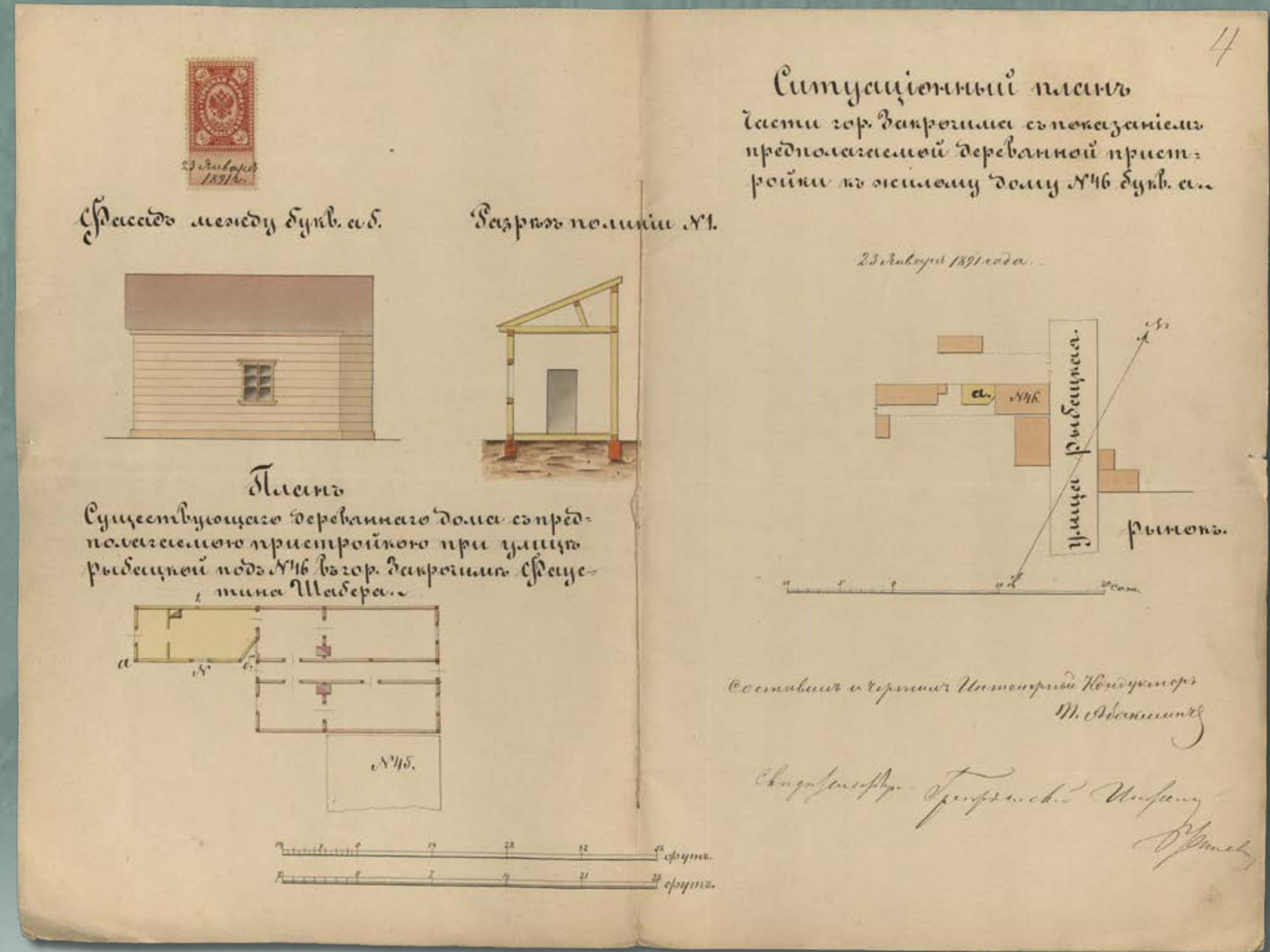
Projekt drewnianej przybudówki do domu mieszkalnego w nieruchomości numer 46 przy ulicy Rybackiej w Zakroczymiu, wł. Faustyn Szaber, 1891 rok (źródło: Archiwum Państwowe w Płocku, Płocki Rząd Gubernialny, sygn. 3218, k. 4)
