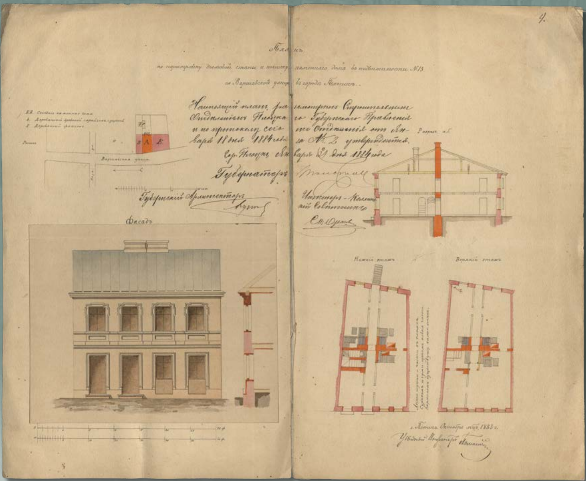
Projekt przebudowy i remontu domu w nieruchomości numer 13 przy ulicy Warszawskiej w Płońsku, wł. Josel Ciechanowski, 1883 rok (źródło: Archiwum Państwowe w Płocku, Płocki Rząd Gubernialny, sygn. 3190, k. 3–4)
