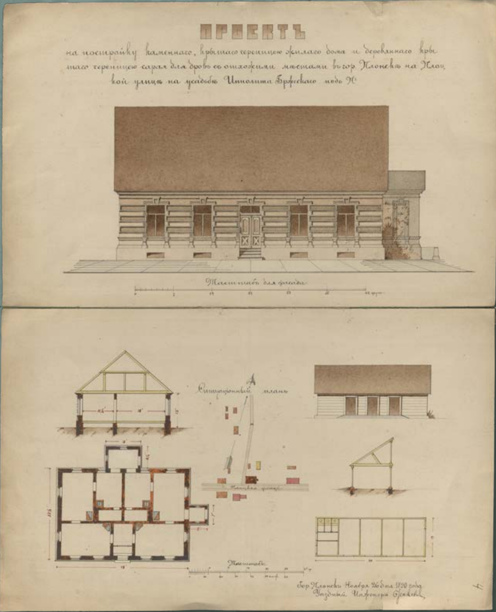
Projekt murowanego krytego dachówką domu mieszkalnego i drewnianego krytego dachówką składu na drwa z ustępami w mieście Płońsku przy ulicy Płockiej, wł. Hipolit Brzeski, 1890 rok (źródło: Archiwum Państwowe w Płocku, Płocki Rząd Gubernialny, sygn. 3217, k. 3–4)
