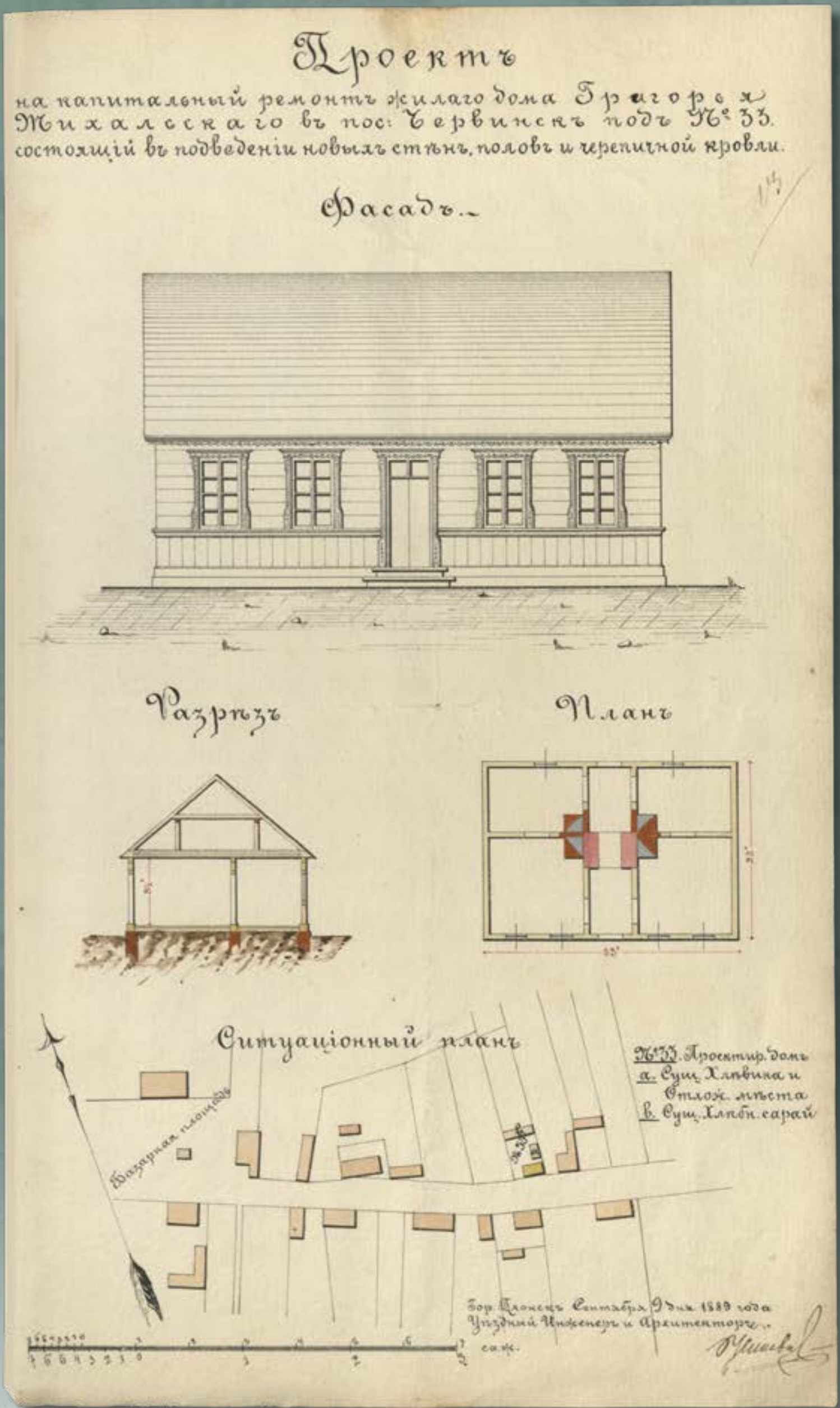
Projekt kapitalnego remontu domu mieszkalnego w nieruchomości pod numerem 33 w Czerwińsku, wł. Grzegorz Zychalski, 1889 rok (źródło: Archiwum Państwowe w Płocku, Płocki Rząd Gubernialny, sygn. 3215, k. 13)
