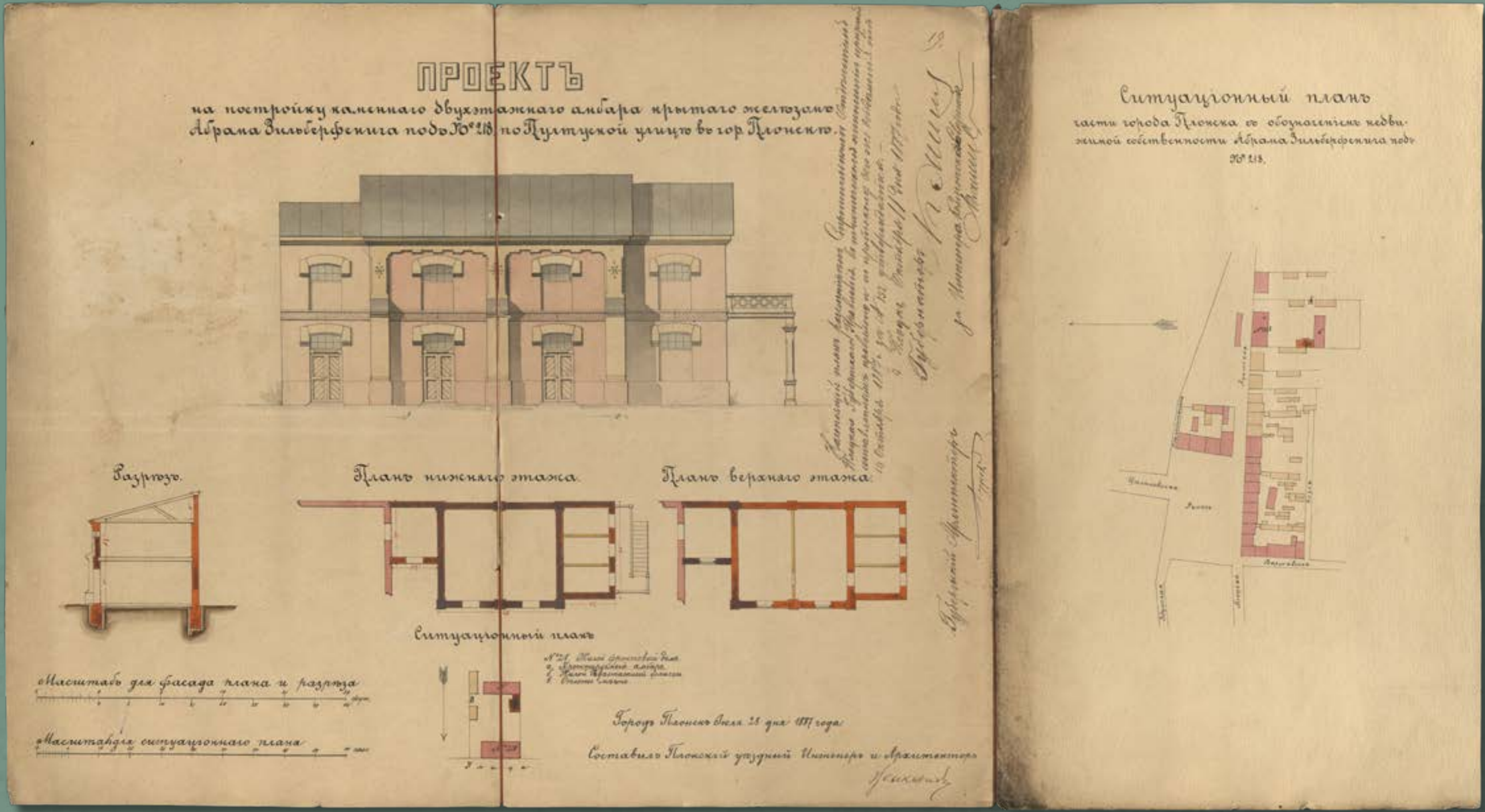
Projekt murowanego dwupiętrowego spichlerza krytego blachą żelazną w nieruchomości numer 218 przy ulicy Pułtuskiej w Płońsku, wł. Abram Zylberfenig, 1887 rok (źródło: Archiwum Państwowe w Płocku, Płocki Rząd Gubernialny, sygn. 3198, k. 19)
