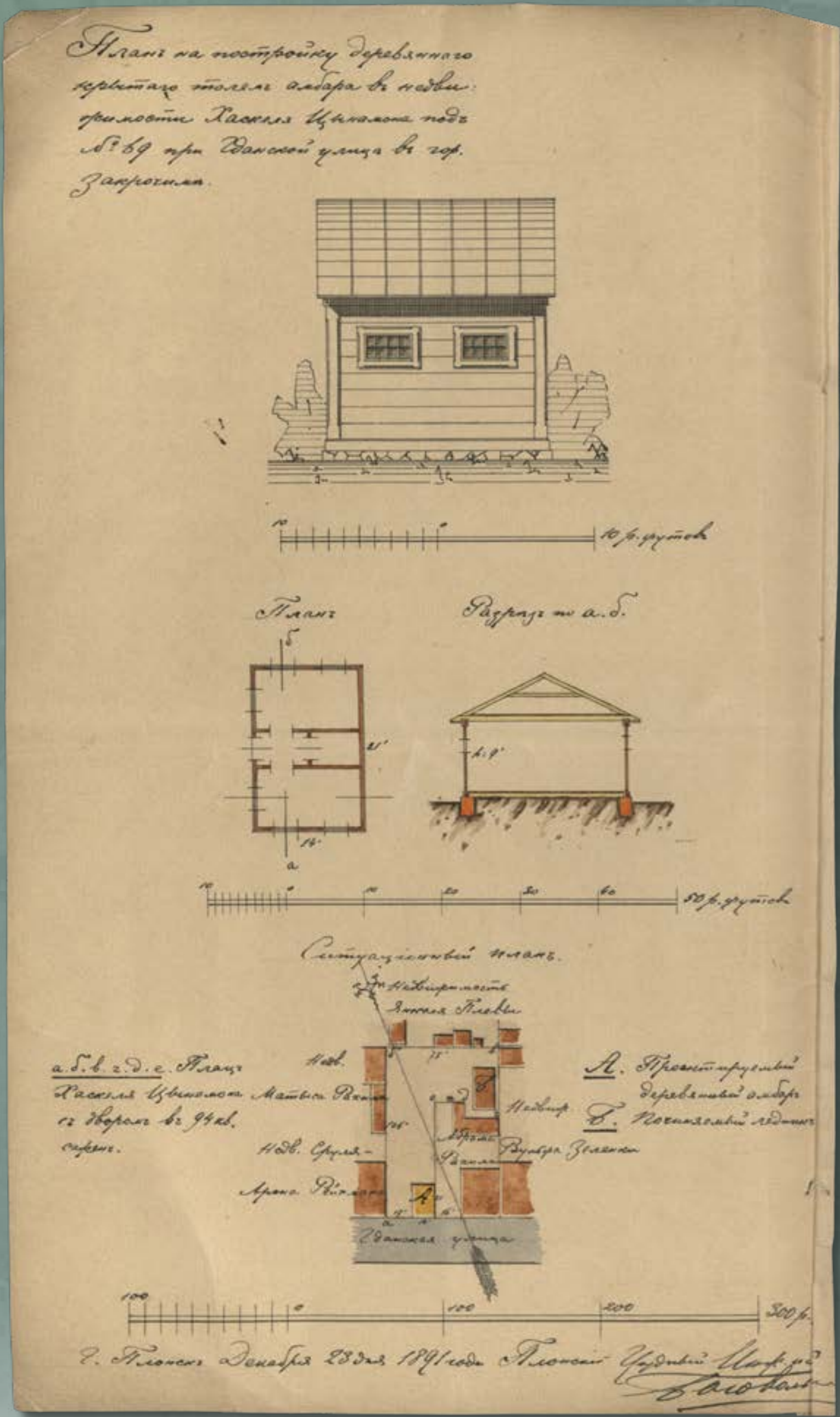
Projekt drewnianego krytego papą spichrza w nieruchomości pod numerem 69 przy ulicy Gdańskiej w Zakroczymiu, wł. Chaskiel Cynamon, 1891 rok (źródło: Archiwum Państwowe w Płocku, Płocki Rząd Gubernialny, sygn. 3222, k. 3)
