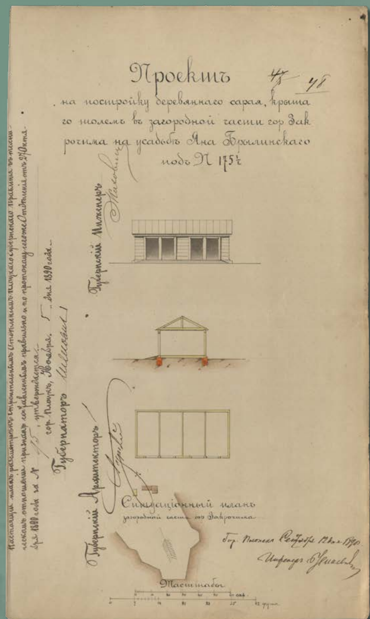
Projekt drewnianej szopy krytej papą na terenie nieruchomości numer 175½ w podmiejskiej części Zakroczymia, wł. Jan Bryliński, 1890 rok (źródło: Archiwum Państwowe w Płocku, Płocki Rząd Gubernialny, sygn. 3214, k. 48)
