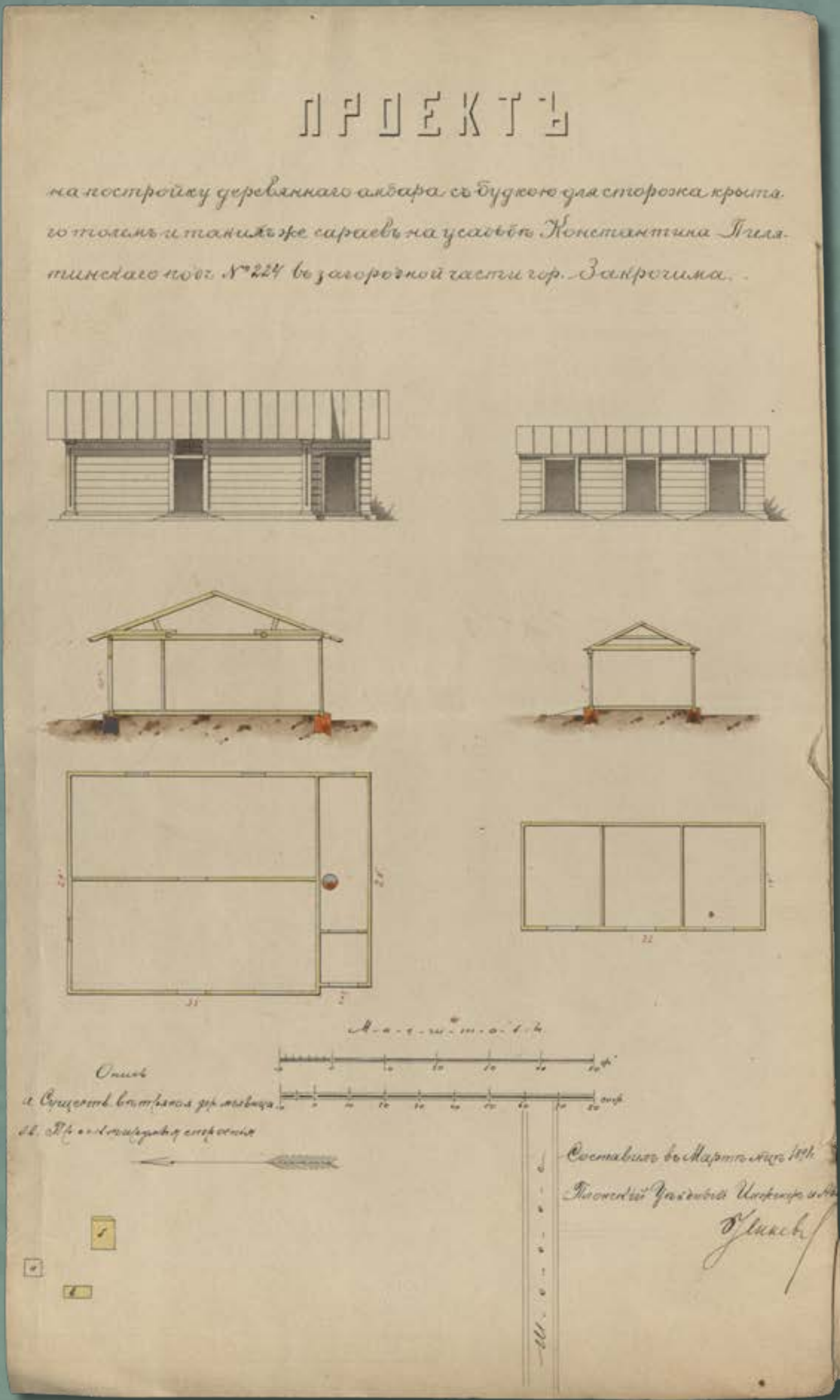
Projekt drewnianego spichrza z budką dla stróża krytego papą w nieruchomości numer 224 w podmiejskiej części Zakroczymia, wł. Konstanty Pilaciński, 1891 rok (źródło: Archiwum Państwowe w Płocku, Płocki Rząd Gubernialny, sygn. 3218, k. 7)
