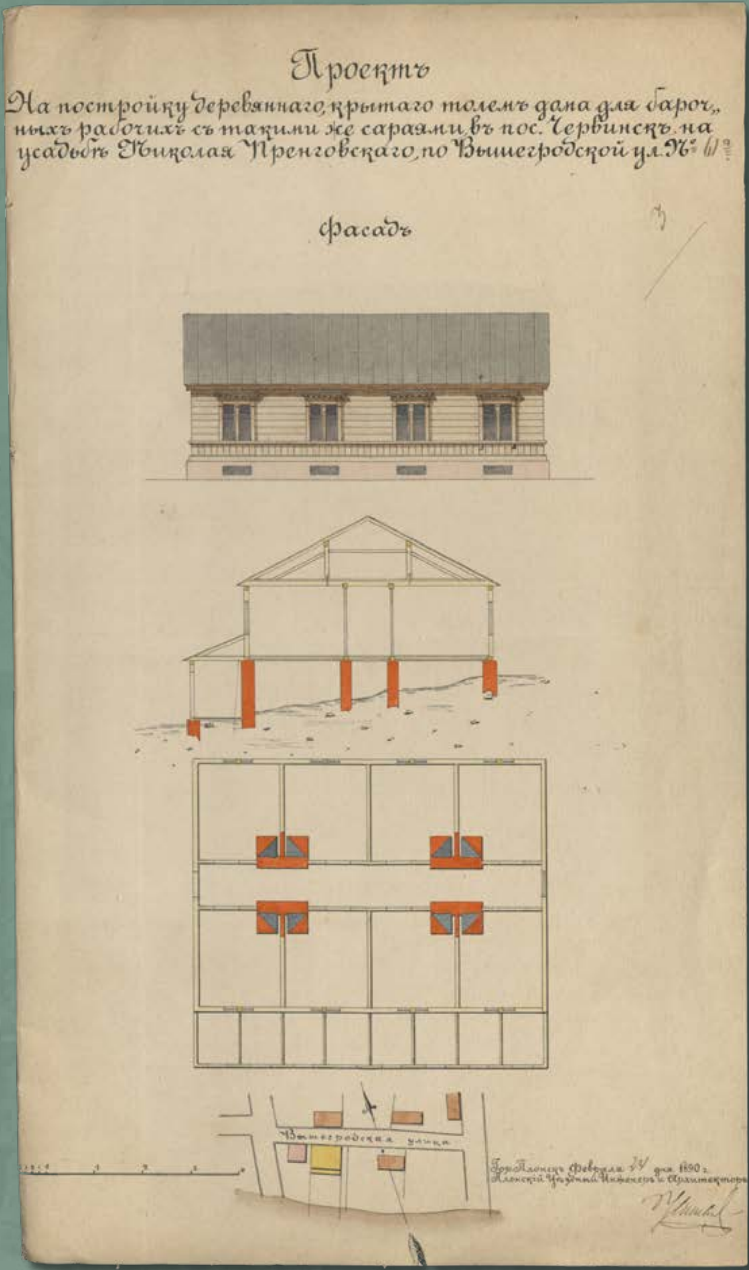
Projekt drewnianego, krytego papą domu mieszkalnego oraz budynków gospodarczych w nieruchomości numer 61a przy ulicy Wyszogrodzkiej w Czerwińsku, wł. Mikołaj Pręgowski, 1890 rok (źródło: Archiwum Państwowe w Płocku, Płocki Rząd Gubernialny, sygn. 3215, k. 3)
