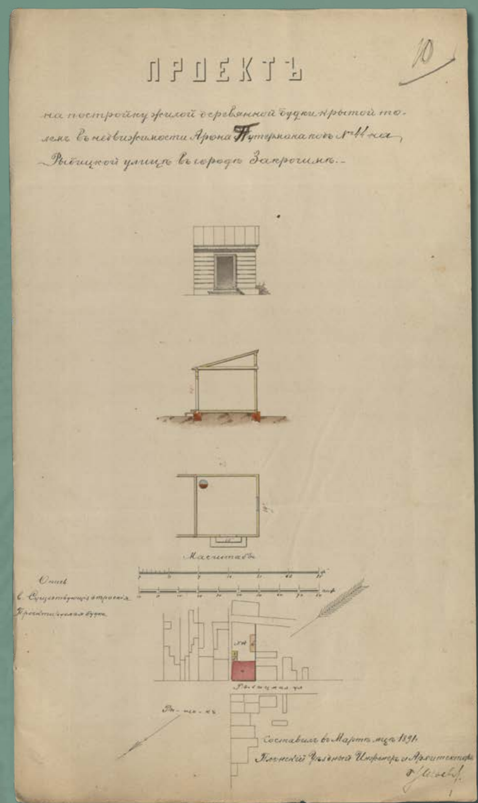
Projekt drewnianej budki mieszkalnej krytej papą w nieruchomości numer 44 przy ulicy Rybackiej w Zakroczymiu, wł. Aron Puterman, 1891 rok (źródło: Archiwum Państwowe w Płocku, Płocki Rząd Gubernialny, sygn. 3218, k. 10)
