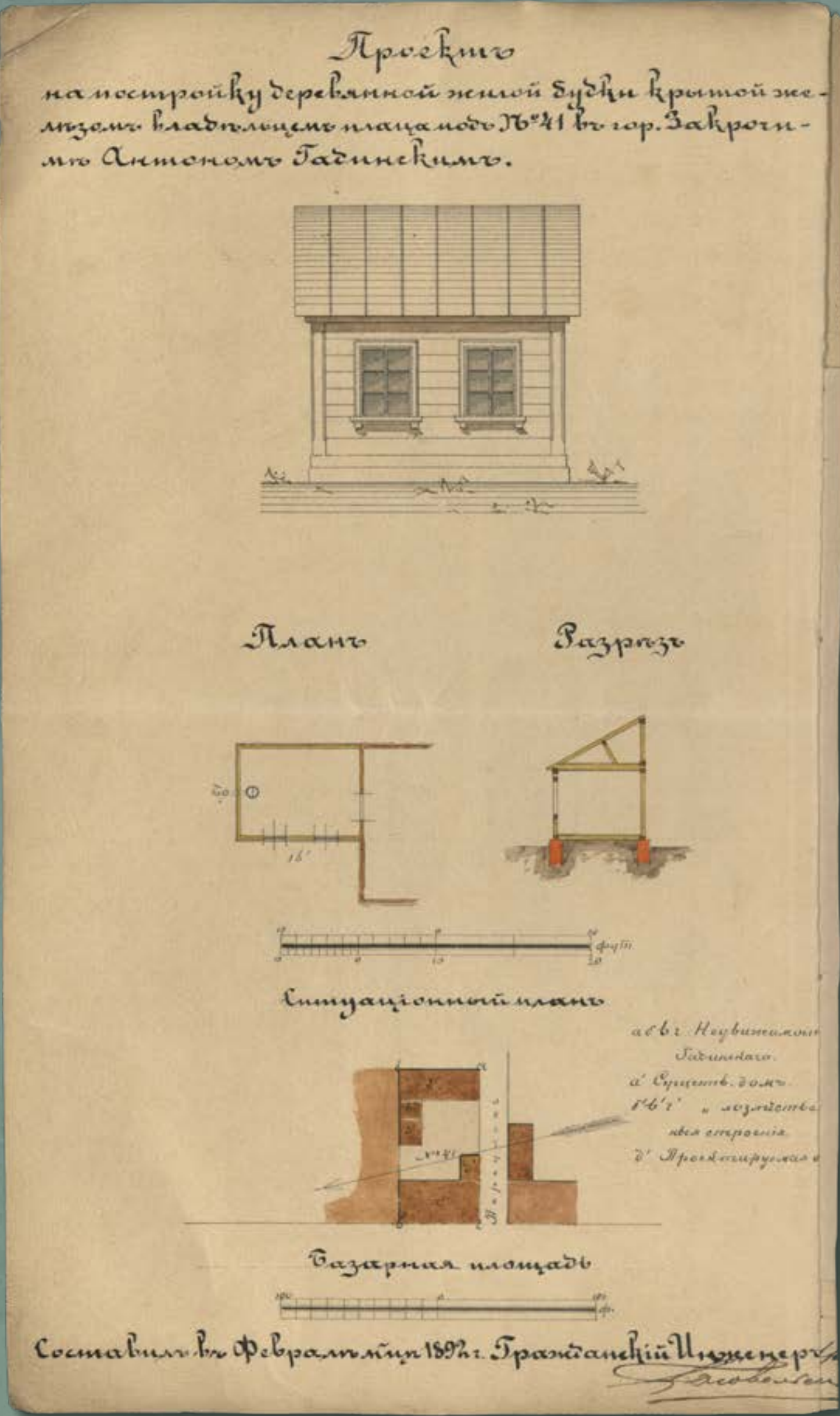
Projekt drewnianej mieszkalnej budki krytej blachą żelazną na placu pod numerem 41 w Zakroczymiu, wł. Antoni Gabiński, 1892 rok (źródło: Archiwum Państwowe w Płocku, Płocki Rząd Gubernialny, sygn. 3222, k. 6)
