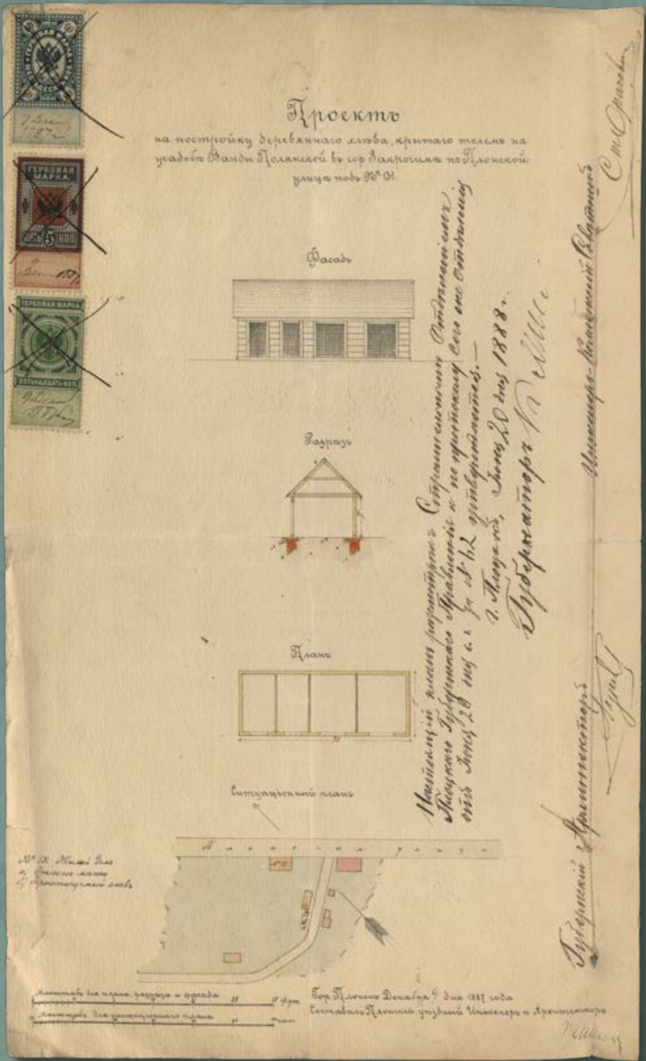
Projekt drewnianego chlewu krytego papą w nieruchomości pod numerem 131 przy ulicy Płockiej w Zakroczymiu, wł. Wanda Polańska, 1887 rok (źródło: Archiwum Państwowe w Płocku, Płocki Rząd Gubernialny, sygn. 3201)
