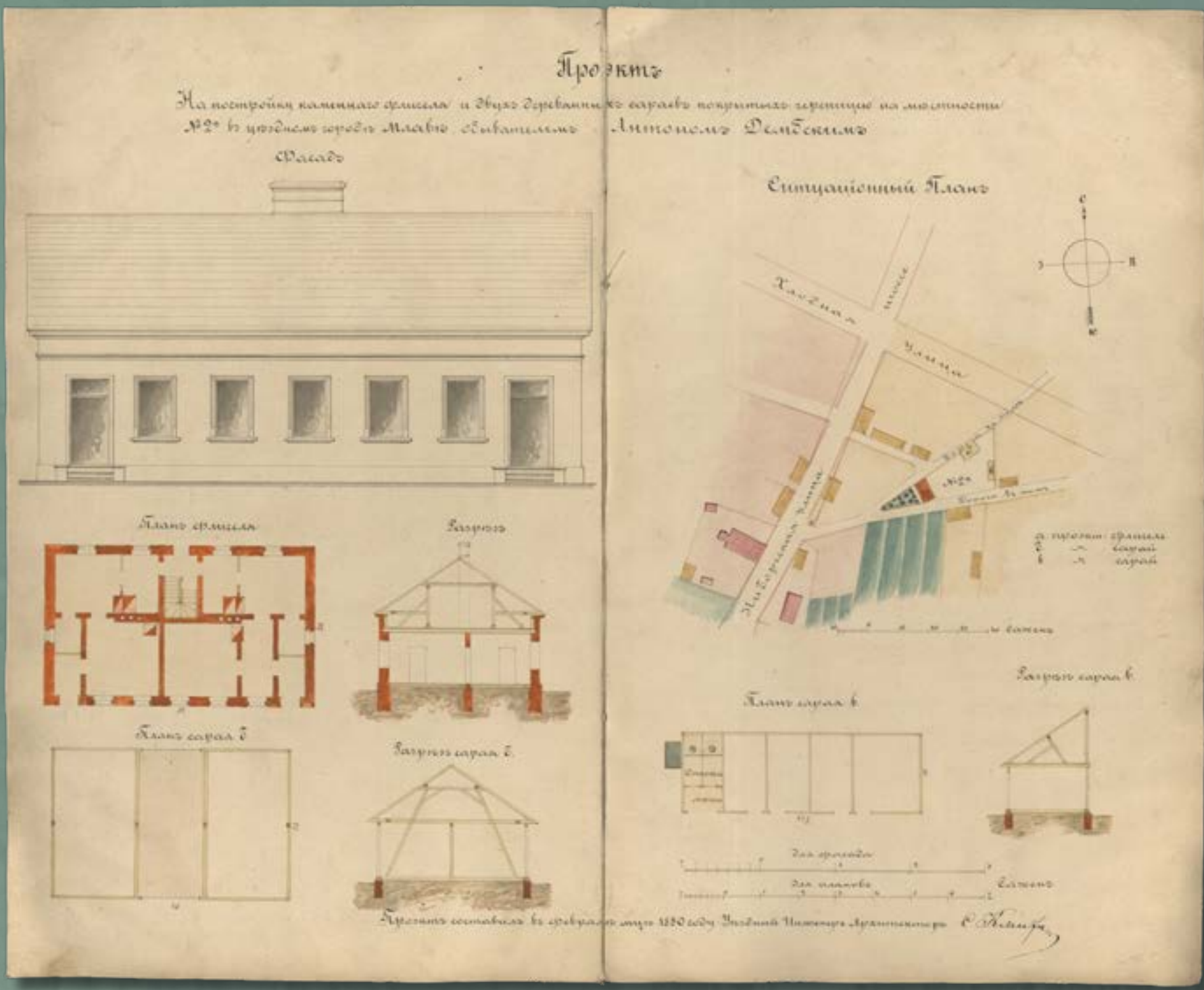
Projekt murowanej oficyny i dwóch drewnianych szop krytych dachówką w nieruchomości numer 2a w Mławie, wł. Antoni Dembski, 1880 rok (źródło: Archiwum Państwowe w Płocku, Płocki Rząd Gubernialny, sygn. 3160, k. 6)
