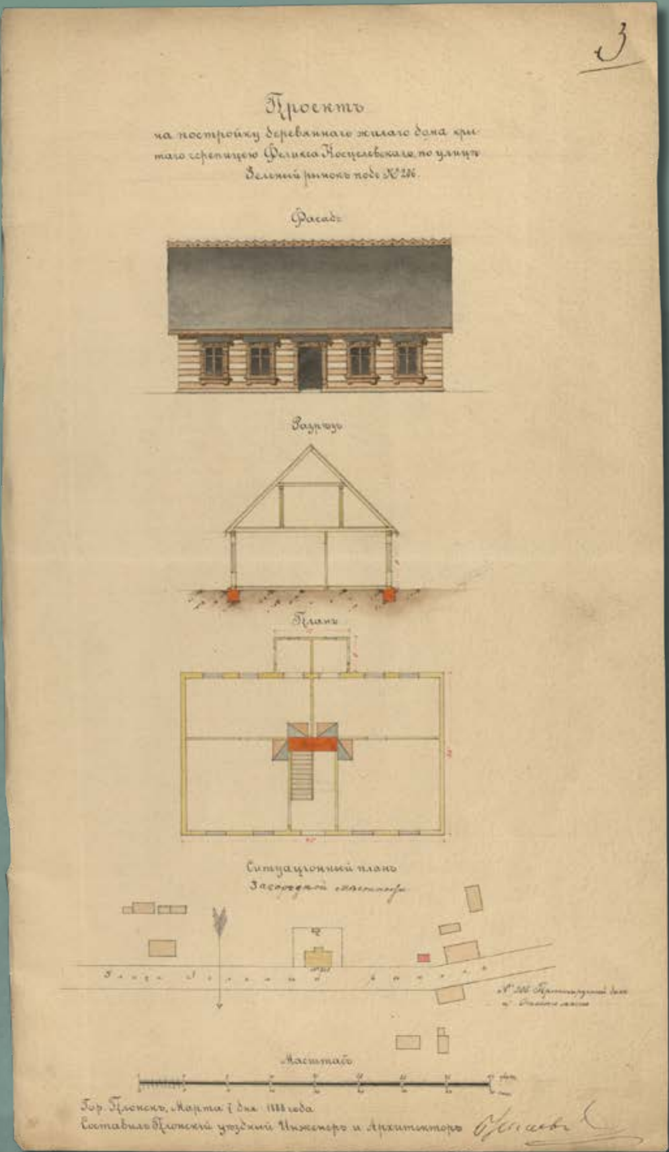
Projekt drewnianego domu mieszkalnego krytego dachówką w nieruchomości numer 206 przy Zielonym Rynku, wł. Feliks Kościelewski, 1888 rok (źródło: Archiwum Państwowe w Płocku, Płocki Rząd Gubernialny, sygn. 3204, k. 3)
