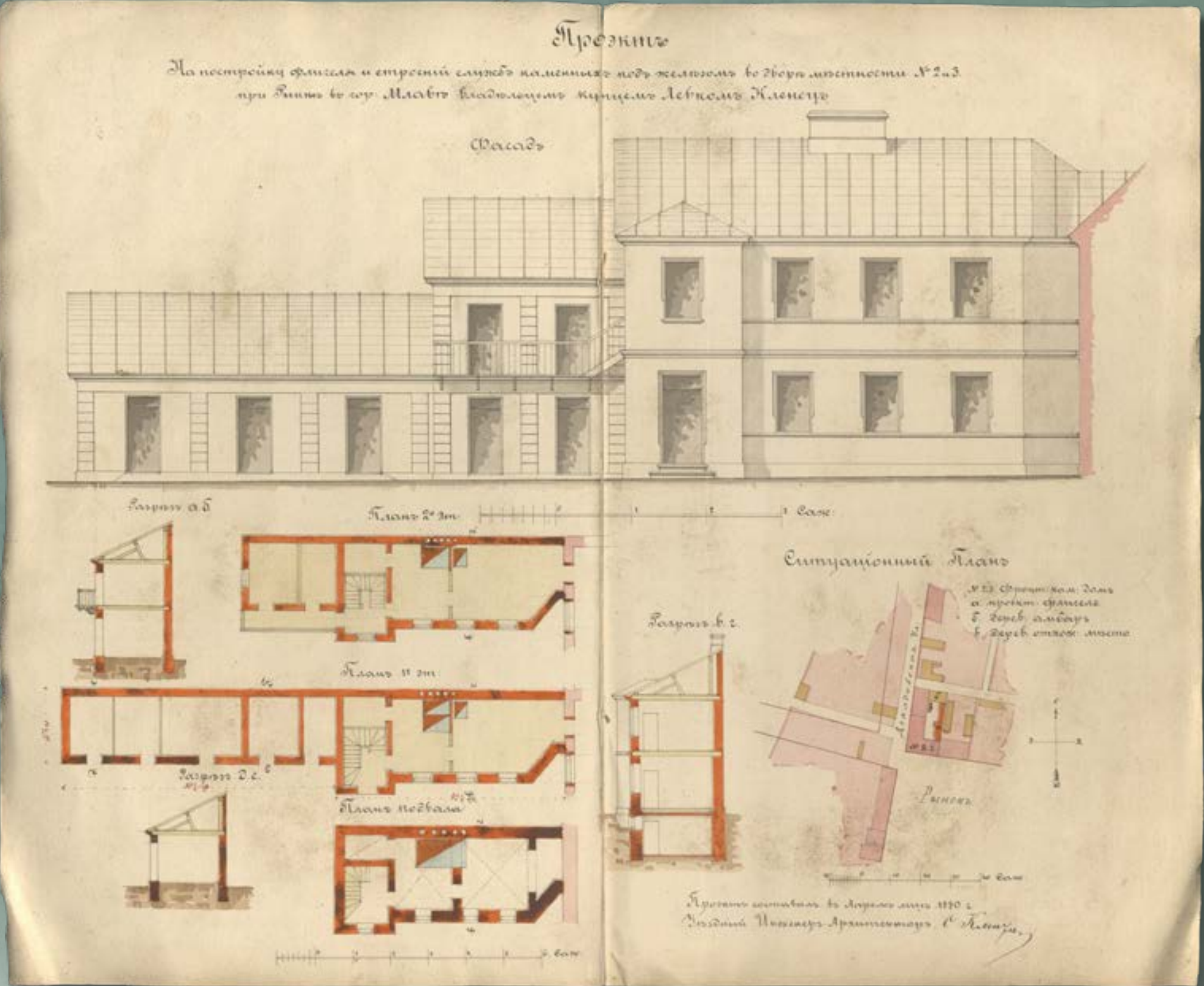
Projekt murowanej oficyny krytej blachą żelazną oraz budynku dla służby w podwórzu nieruchomości numer 2 i 3 przy Rynku w Mławie, wł. Lewek Kleniec, 1880 rok (źródło: Archiwum Państwowe w Płocku, Płocki Rząd Gubernialny, sygn. 3160, k. 15)
