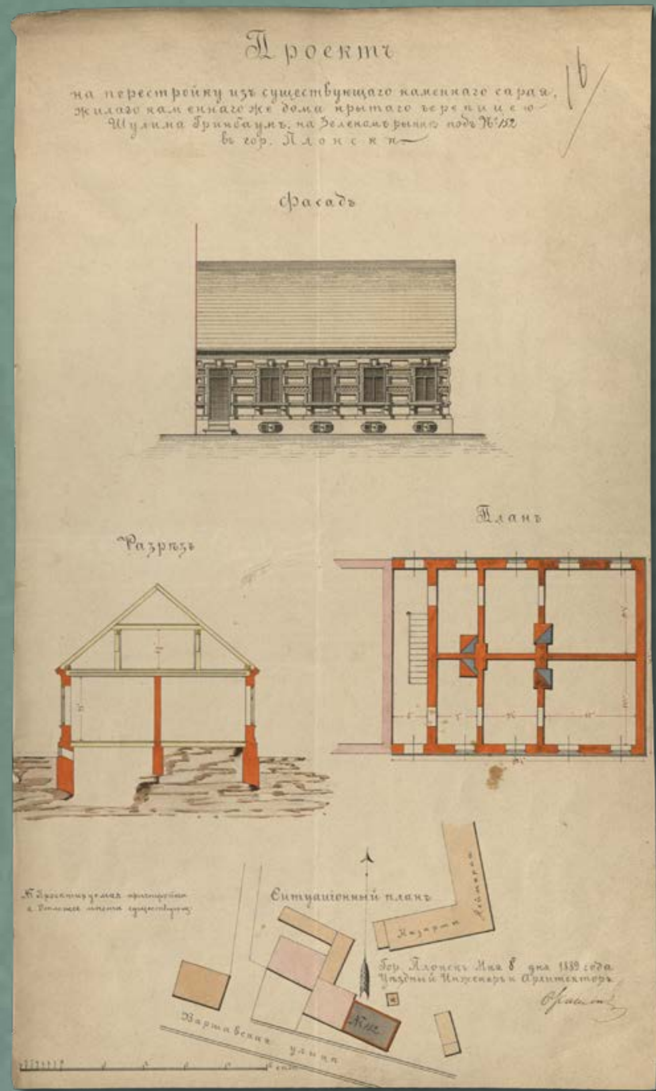
Projekt przebudowy murowanej szopy na murowany dom mieszkalny kryty dachówką w nieruchomości numer 152 przy Zielonym Rynku, wł. Szulim Grynbaum, 1889 rok (źródło: Archiwum Państwowe w Płocku, Płocki Rząd Gubernialny, sygn. 3206, k. 16)
