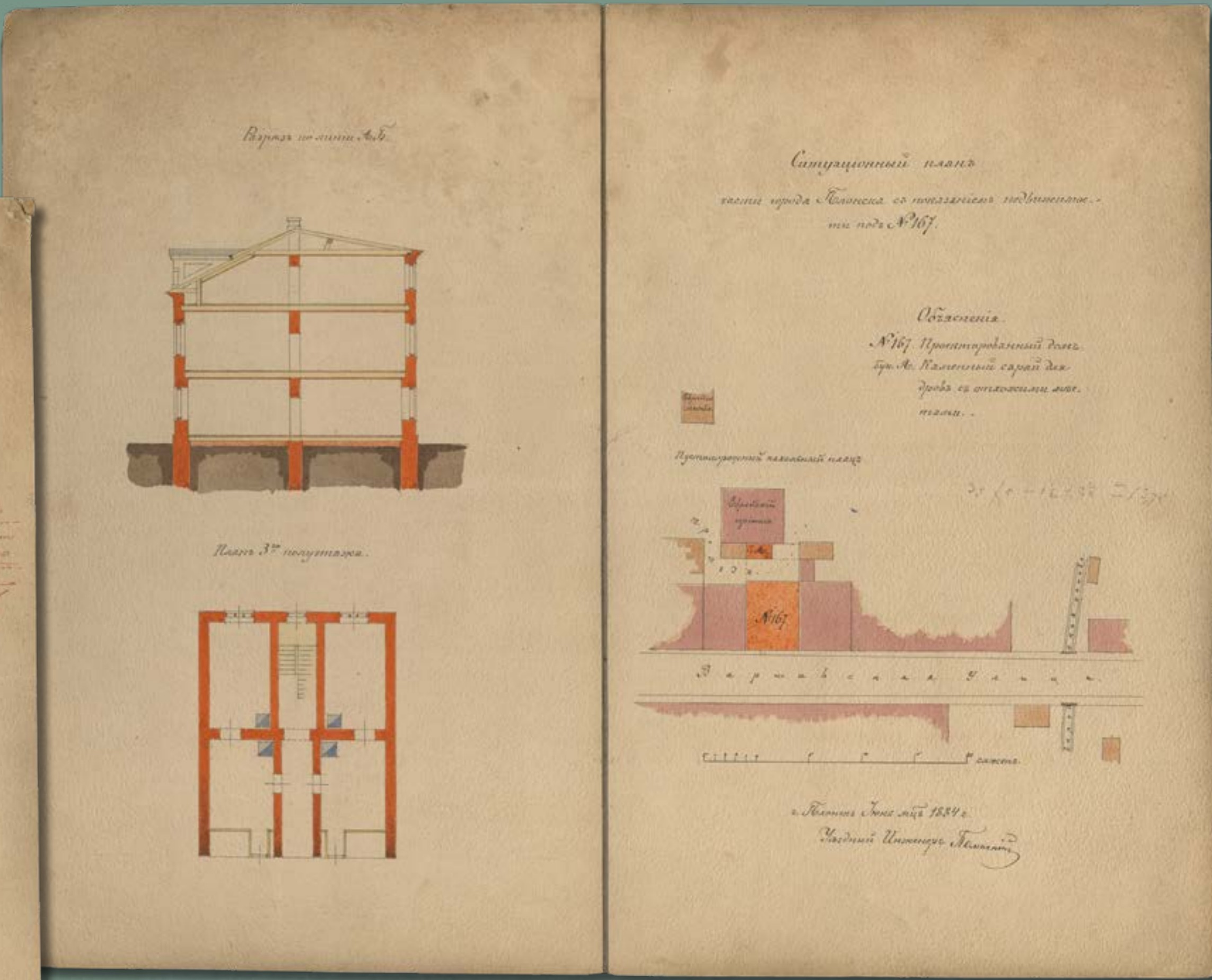
Projekt murowanego frontowego domu krytego blachą żelazną w nieruchomości numer 167 przy ulicy Warszawskiej w Płońsku, wł. Pinkus Jagodziński, 1884 rok (źródło: Archiwum Państwowe w Płocku, Płocki Rząd Gubernialny, sygn. 3190, k. 30)
