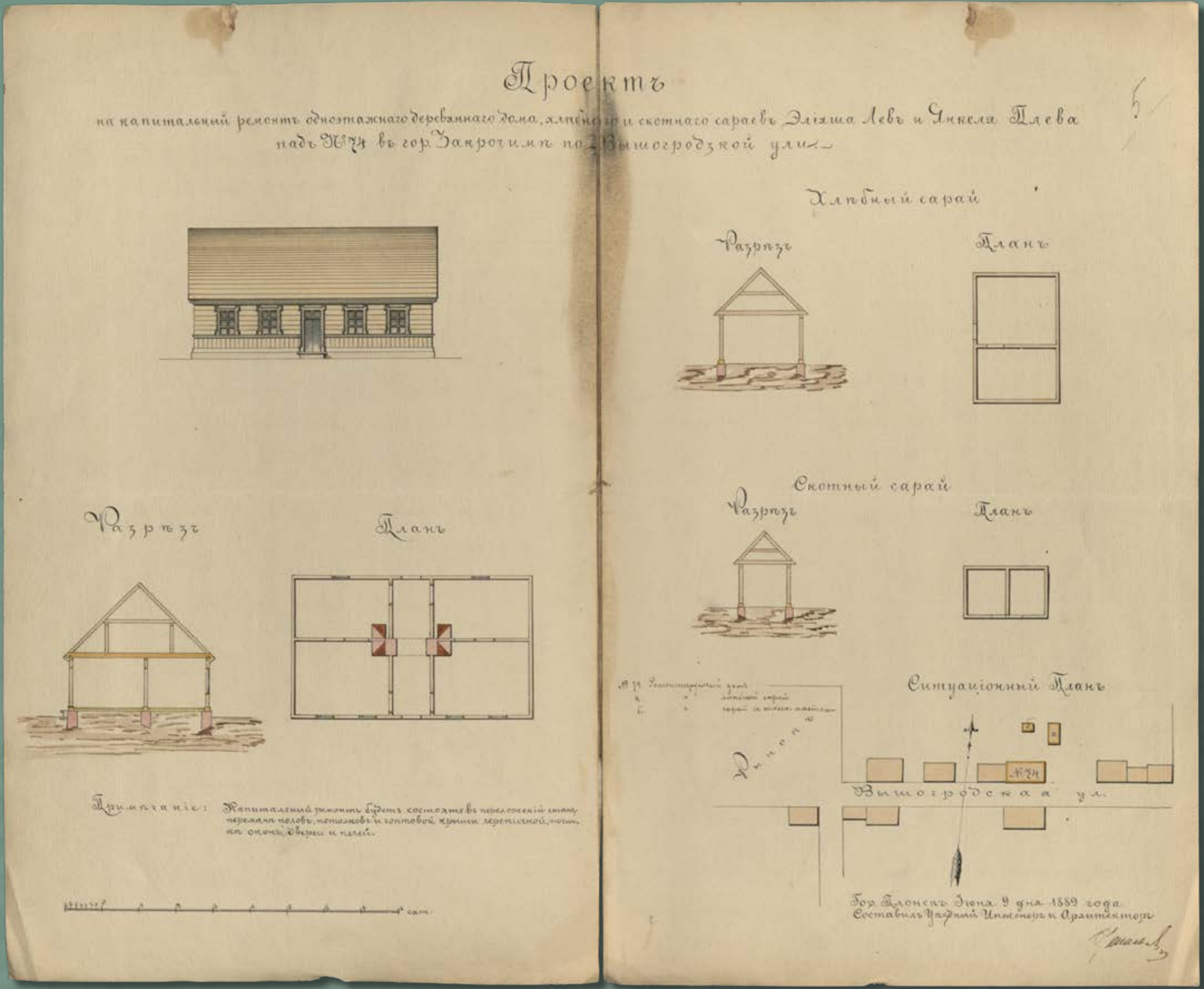
Projekt kapitalnego remontu jednopiętrowego drewnianego domu oraz budynków gospodarczych w nieruchomości pod numerem 74 przy ulicy Wyszogrodzkiej w Zakroczymiu, wł. Eliaz Lew i Jankiel Plew, 1889 rok (źródło: Archiwum Państwowe w Płocku, Płocki Rząd Gubernialny, sygn. 3210, k. 5)
