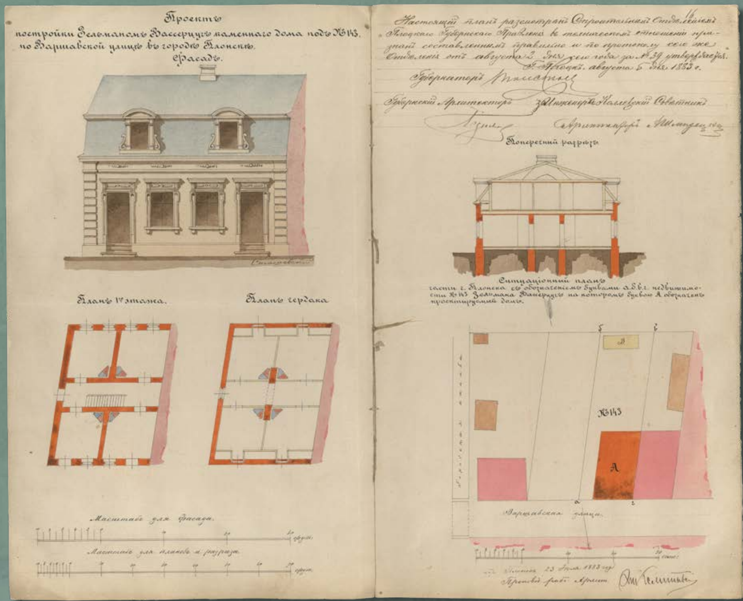
Projekt murowanego domu w nieruchomości numer 143 przy ulicy Warszawskiej, wł. Zelman Wassercug, 1883 rok (źródło: Archiwum Państwowe w Płocku, Płocki Rząd Gubernialny, sygn. 3186, k. 15–16)
