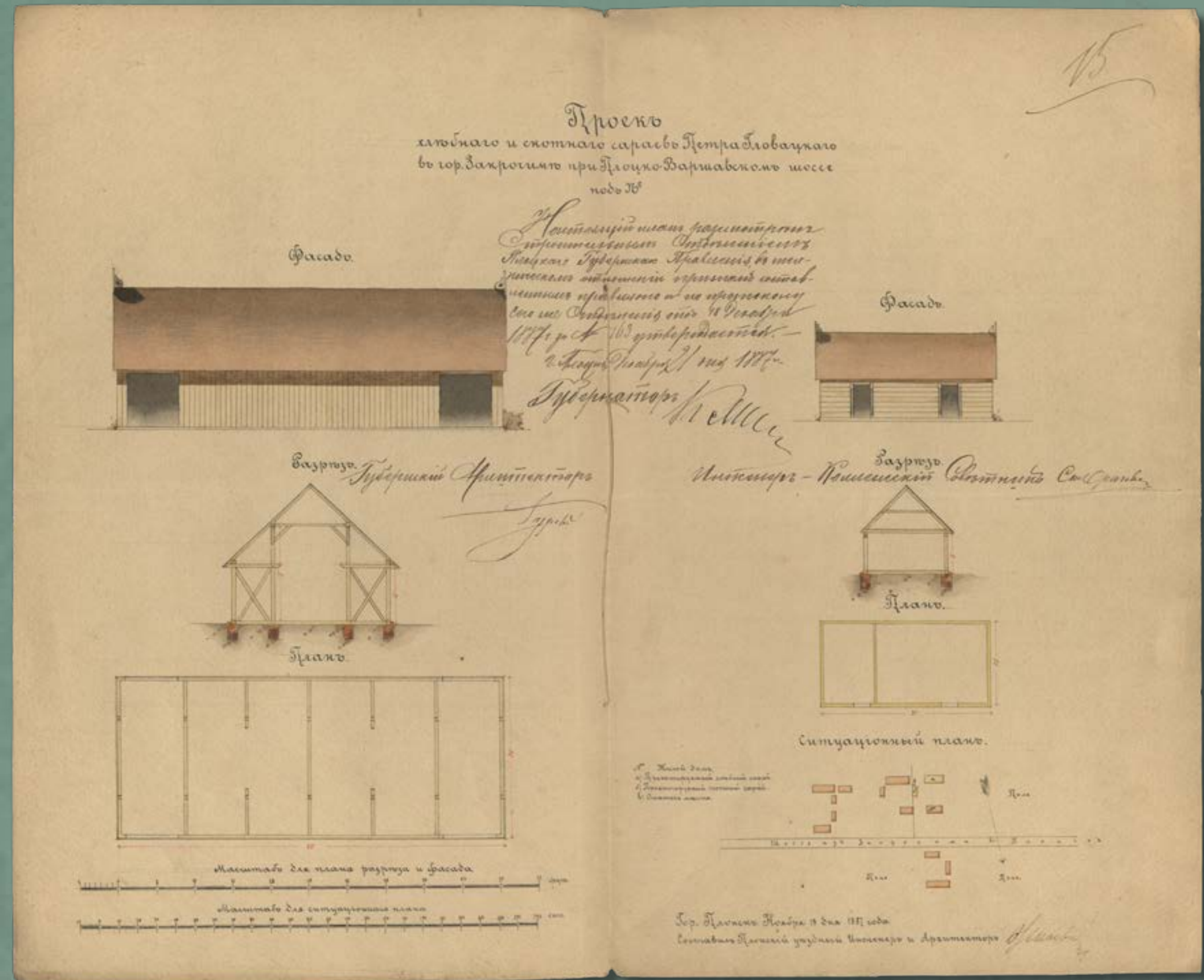
Projekt budynków gospodarczych przy szosie Płocko-Warszawskiej w Zakroczymiu, wł. Piotr Głowacki, 1887 rok (źródło: Archiwum Państwowe w Płocku, Płocki Rząd Gubernialny, sygn. 3200, k. 15)
