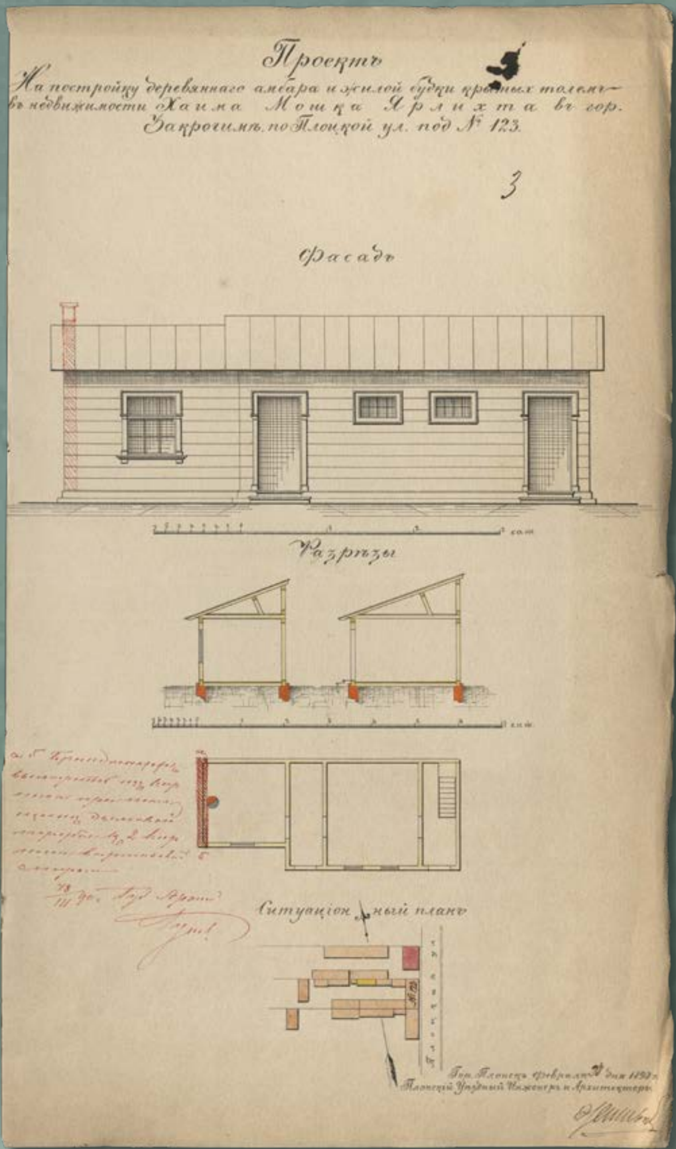
Projekt drewnianego spichrza i mieszkalnej budki krytych papą w nieruchomości numer 123 przy ulicy Płockiej w Zakroczymiu, wł. Chaim Moszek Jarlicht, 1890 rok (źródło: Archiwum Państwowe w Płocku, Płocki Rząd Gubernialny, sygn. 3214, k. 3)
